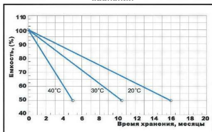
График зависимости ёмкости от времени хранения
