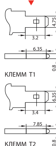
ТИП КЛЕММ
