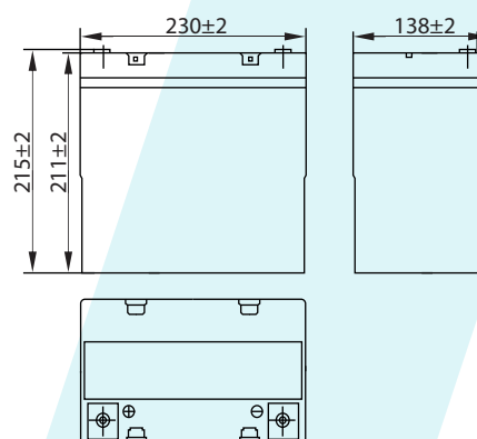
РАЗМЕРЫ
