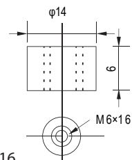
M6 BOLT & NUT
