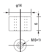
КЛЕММ T9/T16
