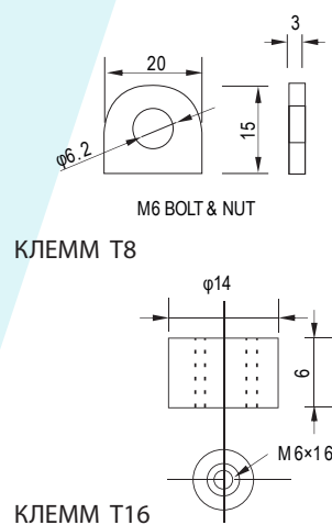
ТИП КЛЕММ
