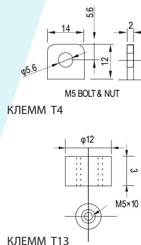
ТИП КЛЕММ
