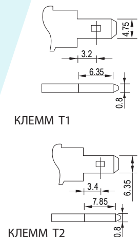
КЛЕММ T2
