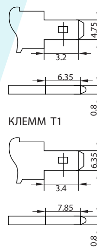
КЛЕММ T2
