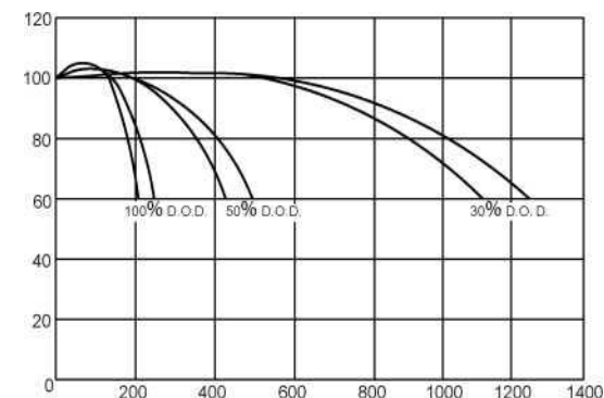
Количество циклов при различной глубине разряда (25 °C)
