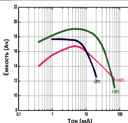
Зависимость ёмкости от тока
