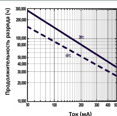
Изменение тока разряда во времени
