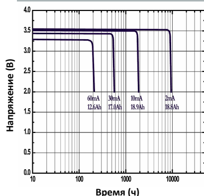
Разрядные характеристики при 20 °C
