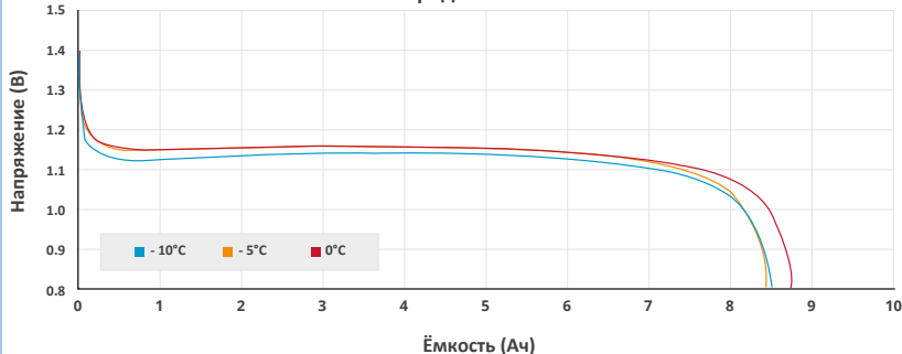
Разрядная ёмкость током 9 А при различных температурах, после быстрого заряда током 4 А
