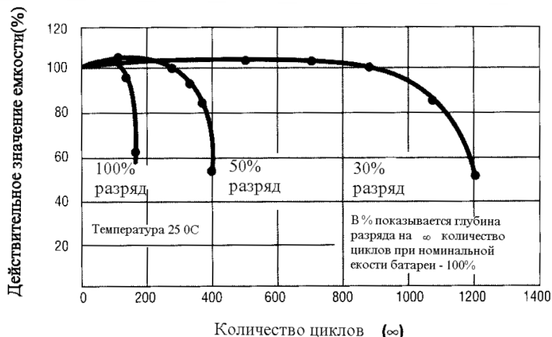
Рисунок 12 – Срок службы при цикличном использовании батареи
