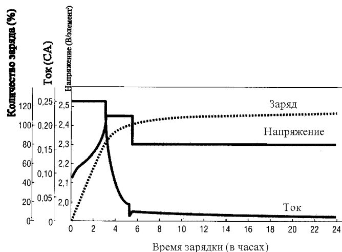
Рисунок 11 – Двухступенчатый заряд батареи 2.45 В/элемент и батареи 2.30 В/элемент при 25°C (77°F)
