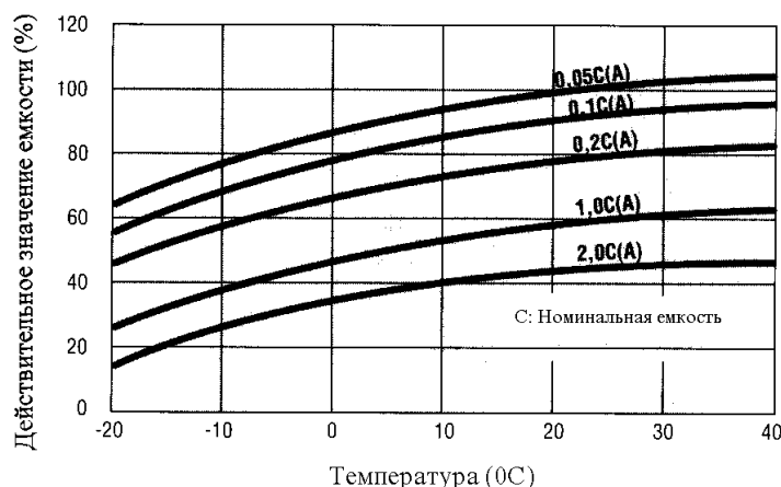
Рисунок 4 Зависимость емкости от температуры
