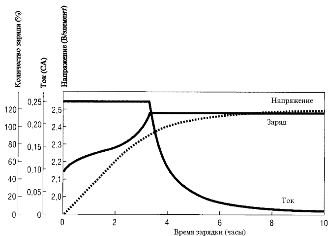
Рисунок 8 – Характеристики заряда при постоянном напряжении (2.45В/элемент, 25°С (77°F))
