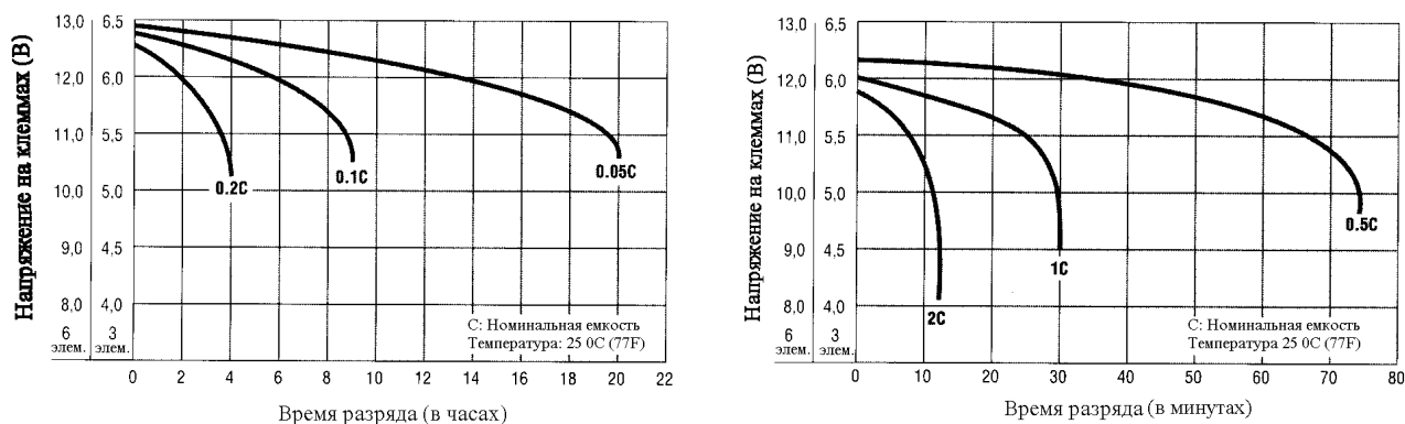
Рисунок 3 – Зависимость времени разряда от тока разряда
