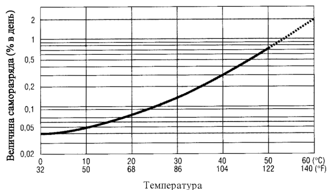
Рисунок 6 – Зависимость величины саморазряда от температуры
