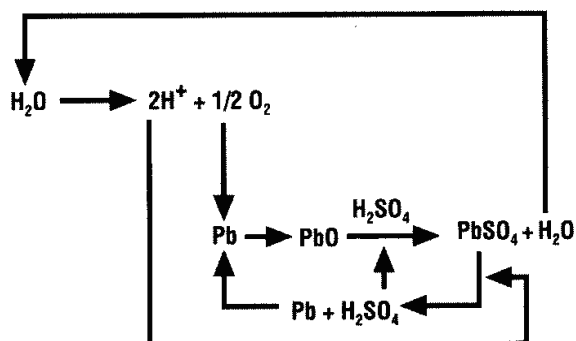
Рисунок 2 Рекомбинационный цикл
