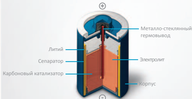
Элемент бобинной конструкции (серия LS)
